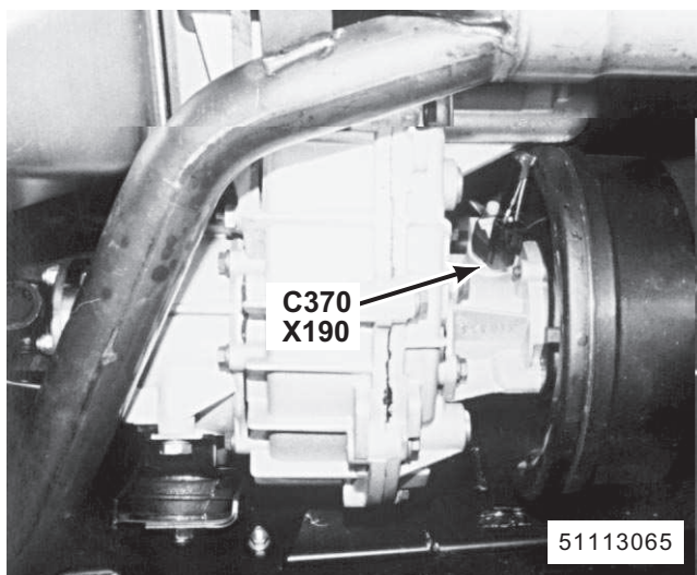
63. onder midden van voertuig X190 Snelheidssensor C370 (3-B)
