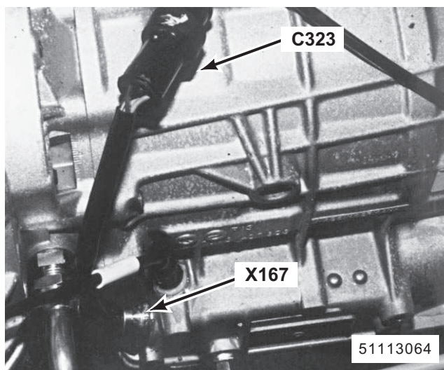
62. linkzijdige transmissie X167 Parkeer-/neutraalstand-schakelaar C323 (5-B)
