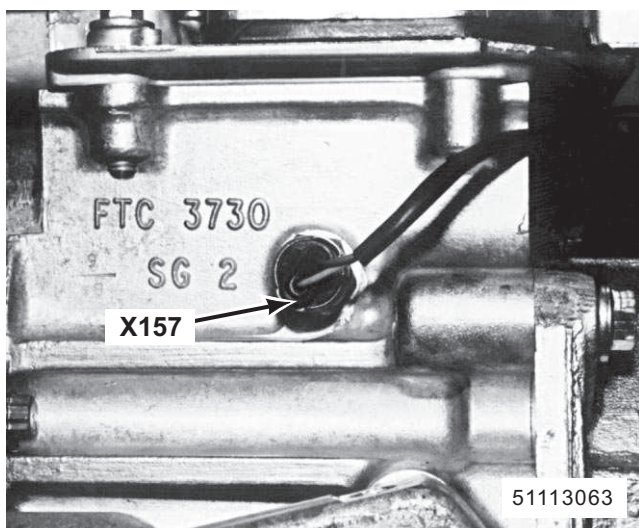
61. linkzijdige transmissie X157 Terugschakelaar
