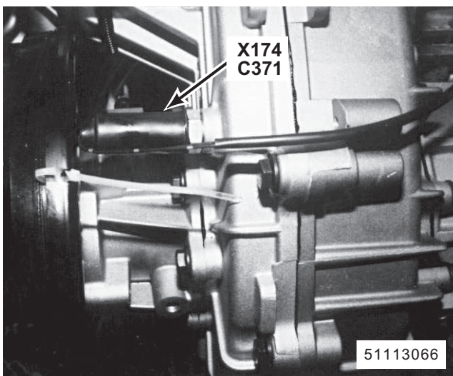
64. rechter bovenkant van tussenbak X174 Olietemperatuurschakelaar tussenbak C371 (2-B)
